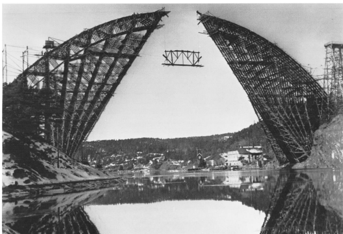
Stillaset til Gamle Svinesunds bro – siste faget heises opp. Foto: Ukjent.
